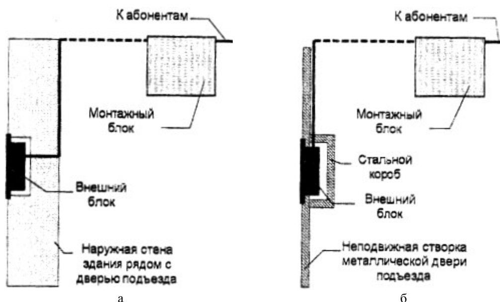
Рисунок 18 - Варианты монтажа блоков подъездного домофона:
