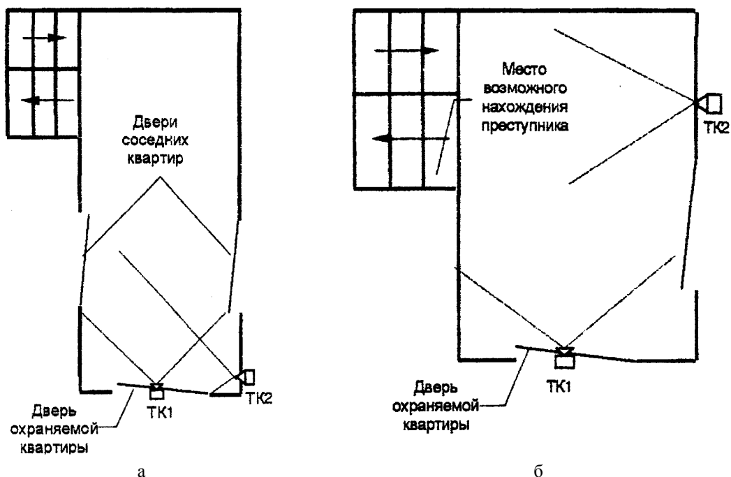
Рисунок 17 - Обзор пространства с помощью дополнительной ТК: а - сбоку от входной двери; б - лестничного пролета
