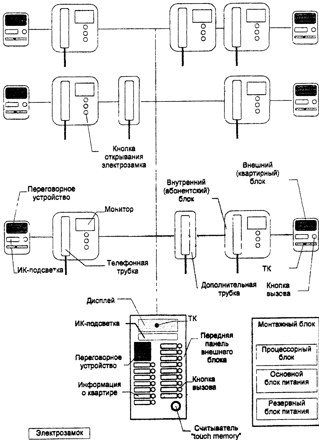
Рисунок 13 - Типовая конфигурация двухуровневого подъездного видеодомофона
