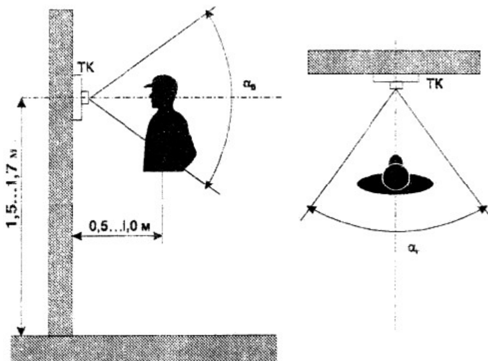
Рисунок 14 - Углы обзора камеры видеодомофона по вертикали ( \alpha_v ) и горизонтали ( \alpha_h )
