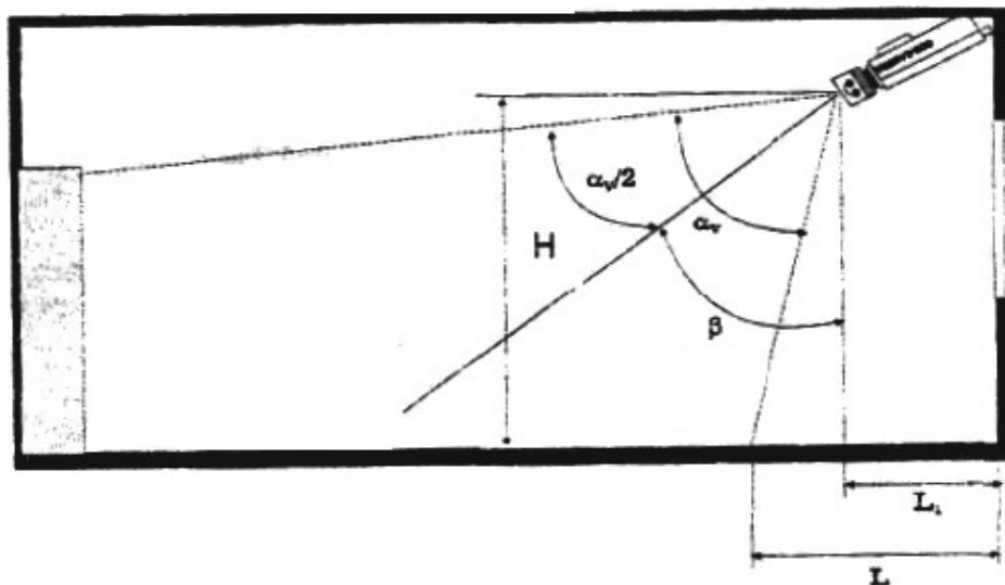
Рисунок 2 - "Мертвая" зона ТК (вид сбоку)
