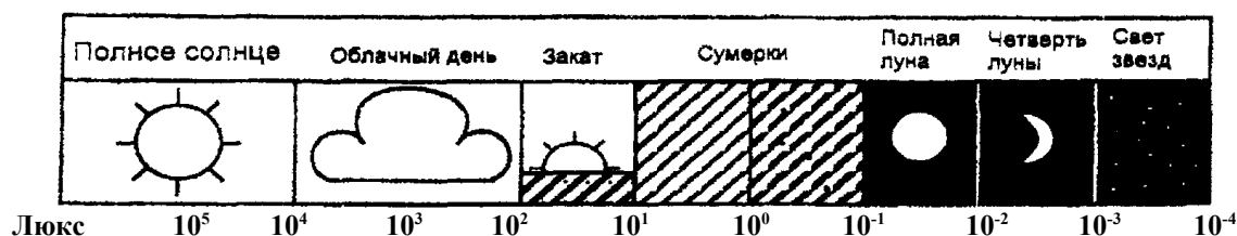
Рисунок 1 - Суточные и. погодные изменения уровней освещенности
