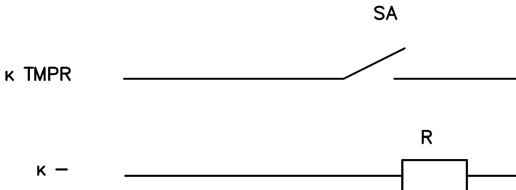
Рис. 15 Схема подключения тампера
