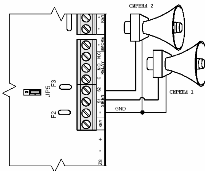
Рис. 10 Подключение сирены типа «горн»
