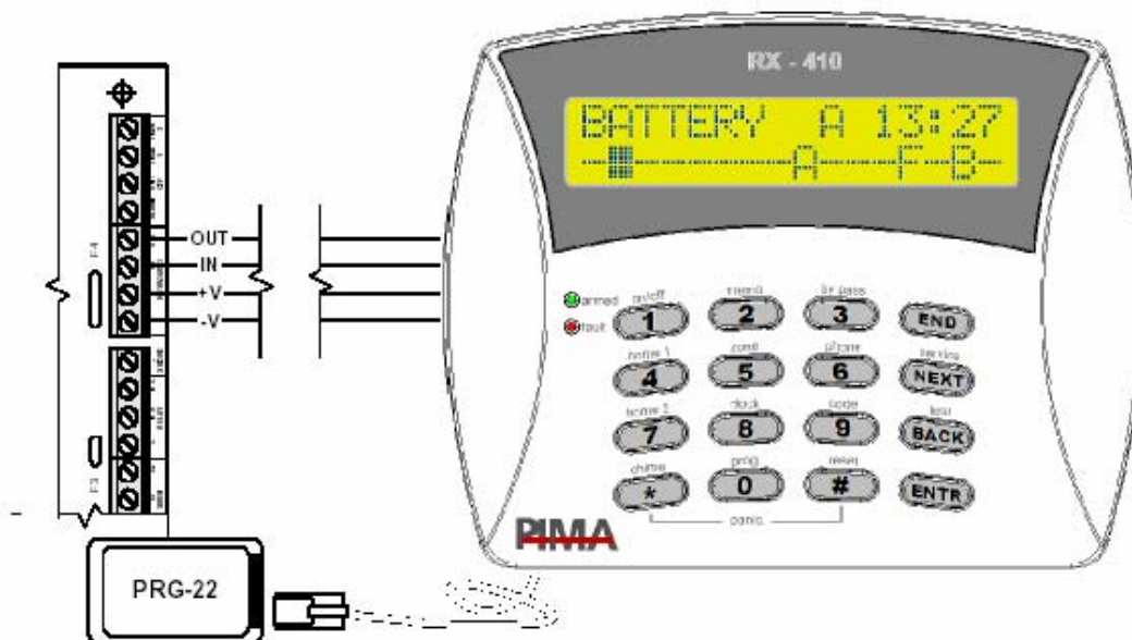
Рис. 23 Подключение программатора
