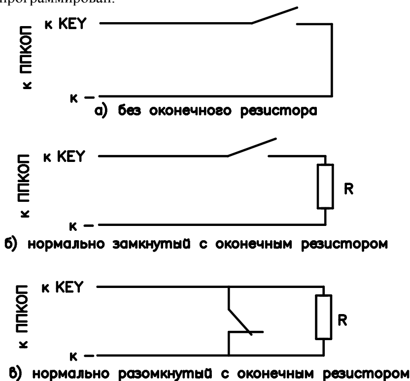
Рис. 9 Способы подключения ключа
