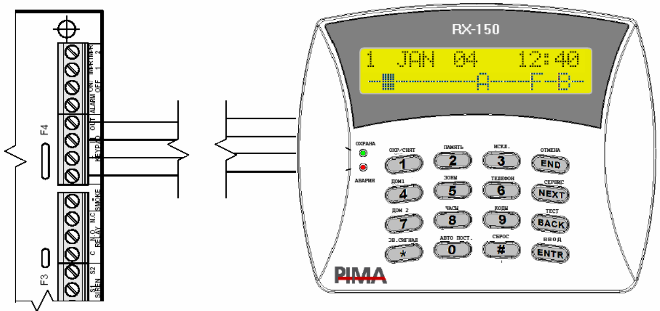
Рис. 12 Подключение клавиатур
