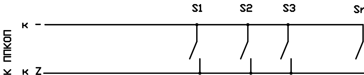
Рис.3 Формирование шлейфа без оконечного резистора из нормально разомкнутых датчиков
