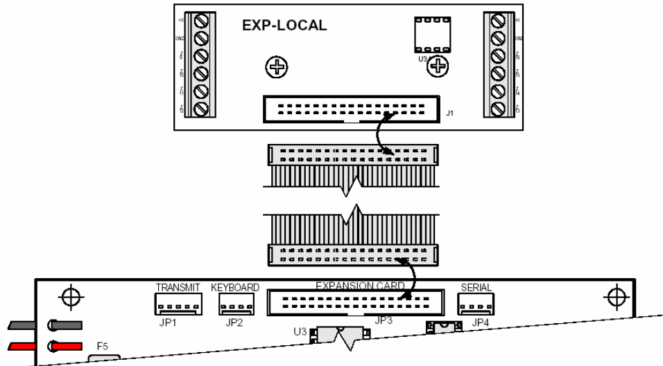
Рис.20 Подключение локального расширителя.
