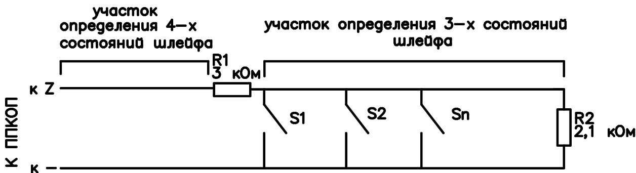
Рис. 46 Участки определения состояний зон
