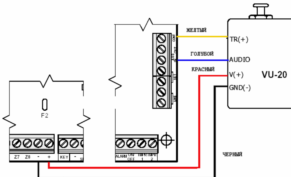
Рис. 18 Подключение голосового блока.
