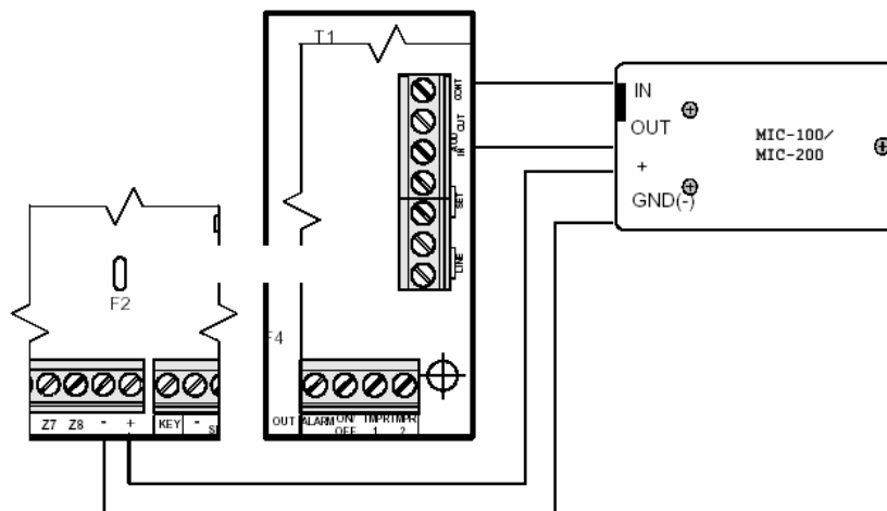
Рис.17 Подключение микрофона
