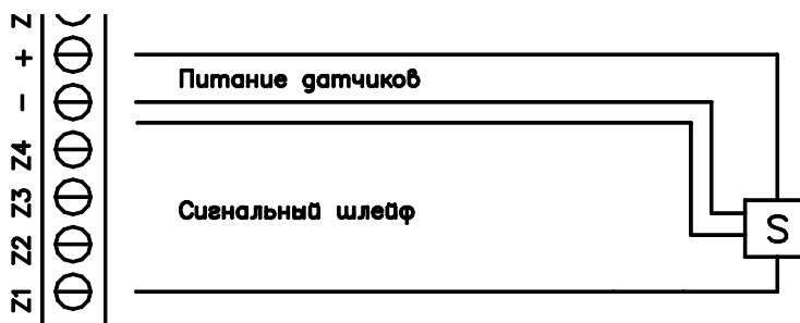
Рис. 2 Подключение датчиков к ППКОП «Hunter-Pro»
