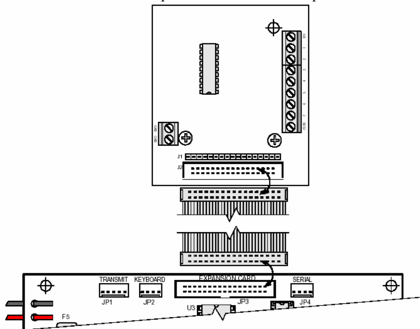
Рис.21 Подключение блока дополнительных выходов.
