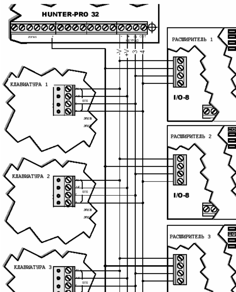
Рис. 14 Подключение расширителей и клавиатур.
