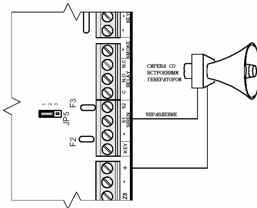
Рис. 11 Подключение сирены с встроенным генератором
