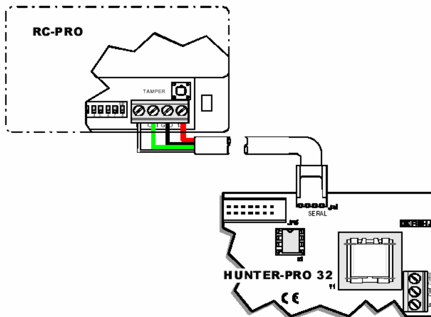
Рис.19 Подключение беспроводного приемника.
