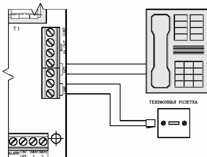
Рис. 16 Подключение телефонной линии и дополнительных устройств
