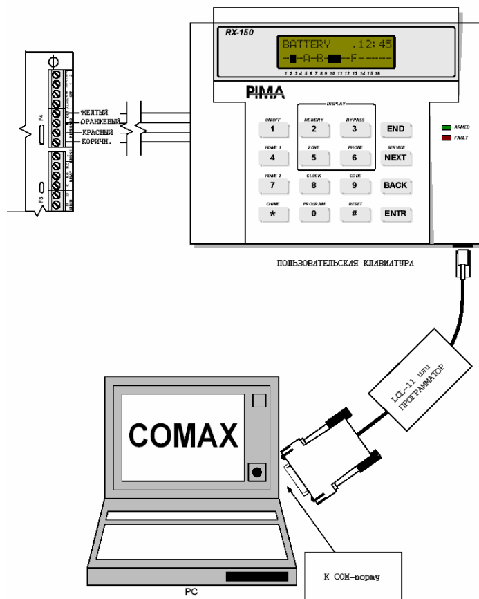
Рис. 24 Подключение для локального программирования.
