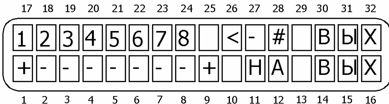
Рис. 38 Установка полярности выходов блока OUT-1000.
