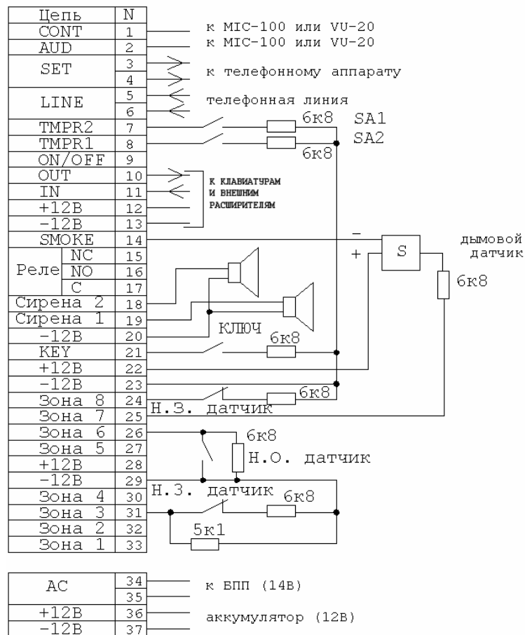
Рис. 22 Типовая схема подключений.
